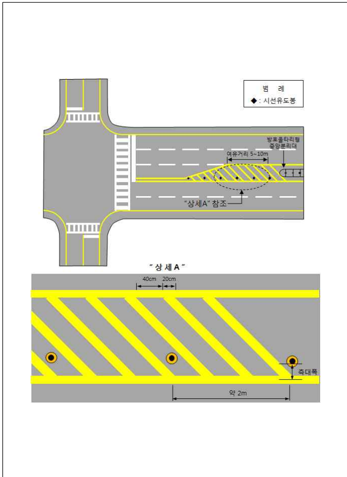
<그림 5.8> 방호울타리형 중앙분리대 전방의 시선유도봉 설치 (교차로)
