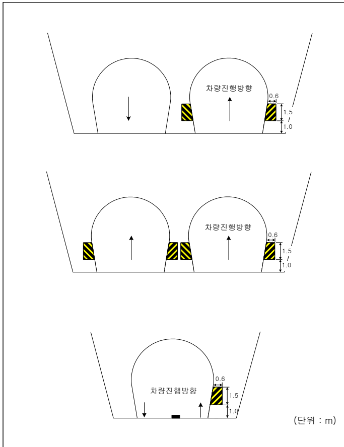
<그림 5.26> 터널 입구의 도색 예
