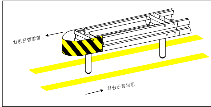
<그림 5.10> 방호울타리형 중앙분리대의 단부 도색 방안
