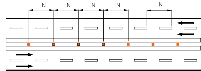
<그림 4.3> 일반적인 직선부에서의 표지병 설치간격
