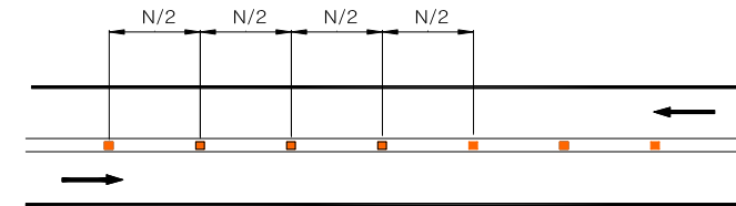
<그림 4.4> 편도 1차로 도로의 표지병 설치간격(부착식)
