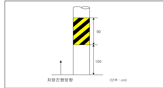
<그림 5.30> 전주 및 기타 구조물의 도색 예
