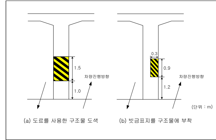
<그림 5.5> 지하차도 기둥에서의 구조물 도색 및 빗금표지 설치
