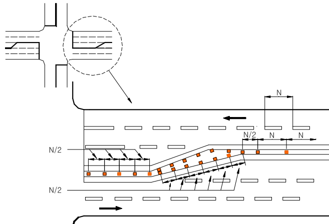
<그림 4.6> 교차로 좌회전 차로 부근의 표지병 설치방법
