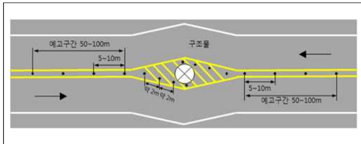
<그림 5.13> 시선유도봉의 설치 방법
