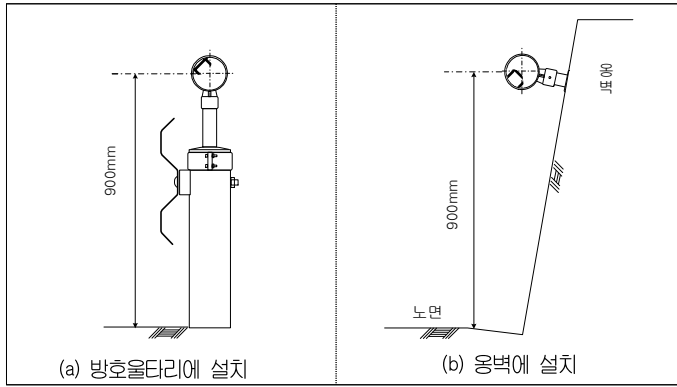
<그림 2.2> 방호울타리, 옹벽에서의 설치 예(원형)
