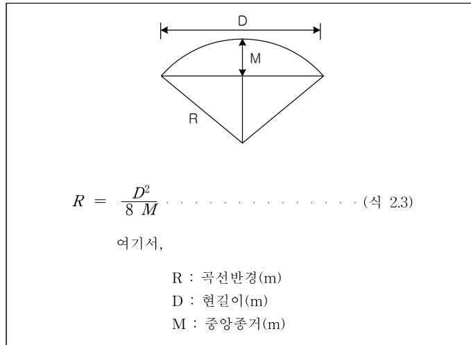
<그림 2.10> 현장에서의 도로 곡선반경 측정
