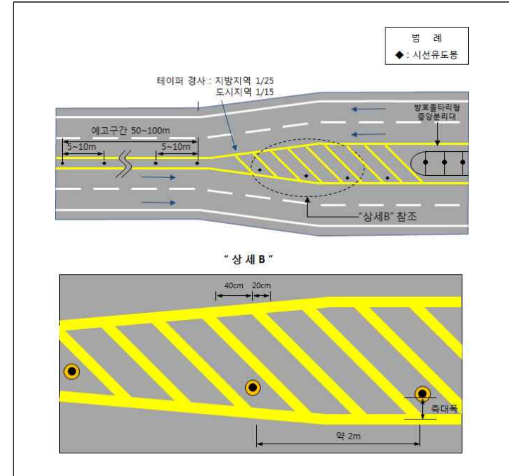
<그림 5.9> 방호울타리형 중앙분리대 전방의 시선유도봉 설치 (단일로)
