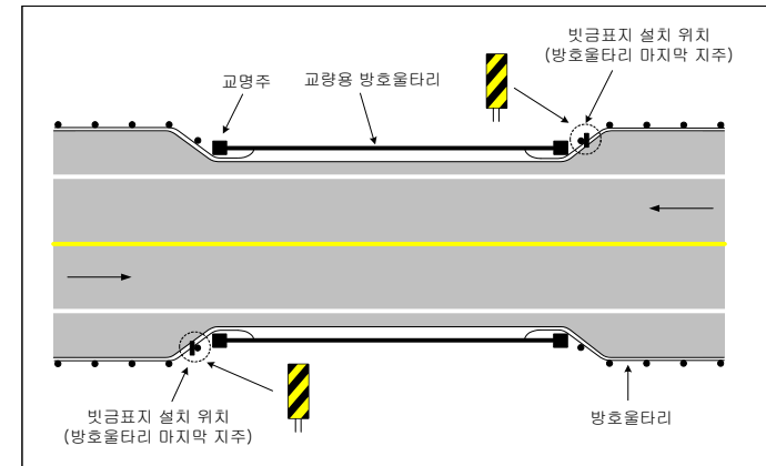
<그림 5.25> 교량 진입부에서의 빗금표지 설치 위치
