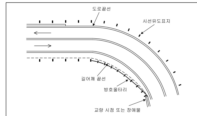
<그림 2.5> 장애물과 시선유도표지의 연계 설치
