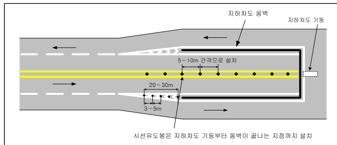
<그림 5.22> 지하차도에서의 시선유도봉 설치 방법
