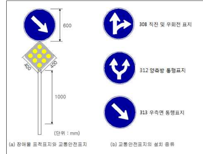
<그림 5.2> 장애물 표적표지의 설치
