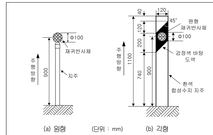
<그림 2.1> 시선유도표지
