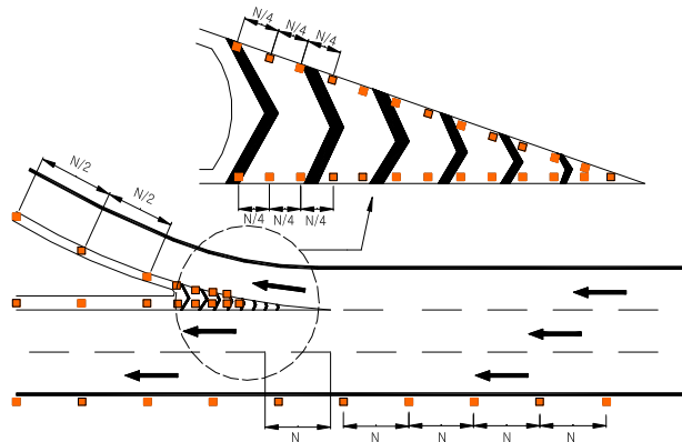
<그림 4.5> 고속도로 진입·출입연결로에서의 표지병 설치방법
