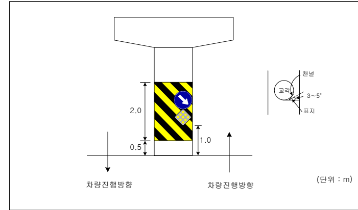
<그림 5.14> 교각의 시인성 향상을 위한 관련 시설의 설치 방법
