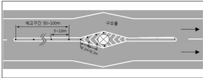
<그림 5.18> 시선유도봉의 설치 방법
