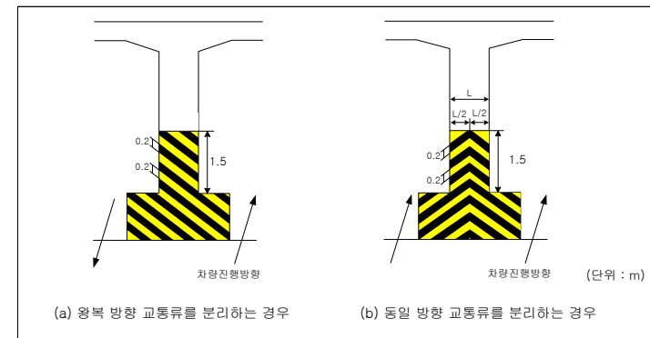
<그림 5.20> 기초가 있는 지하차도의 기둥
