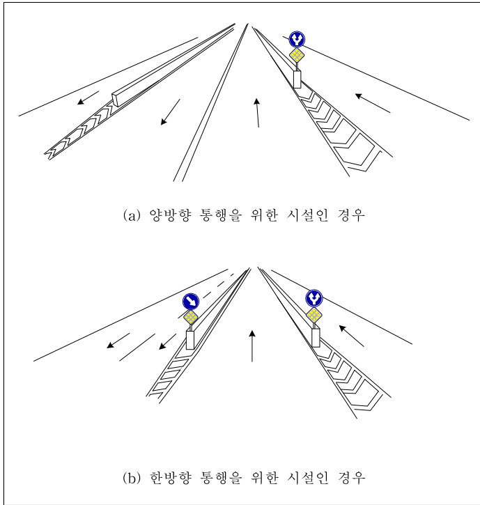
<그림 5.23> 입체교차를 위한 시설 구조물의 단부 처리
