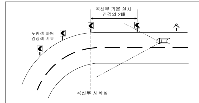
<그림 3.3> 갈매기표지와 교통안전표지의 설치 예
