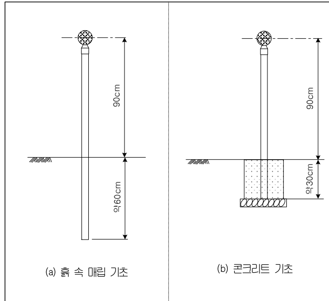
<그림 2.11> 시선유도표지의 기초
