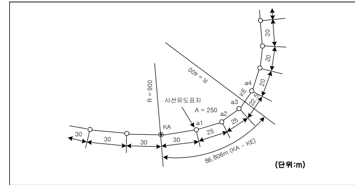
<그림 2.8> 시선유도표지의 설치 (클로소이드구간 사례 II)
