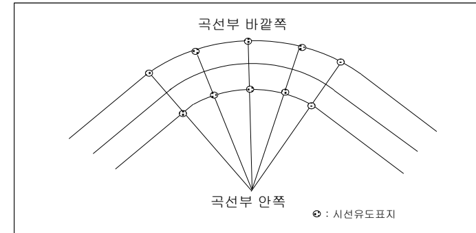
〈그림 2.9〉 곡선부 바깥쪽과 안쪽에서의 설치 방법
