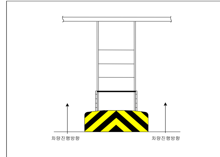
<그림 5.27> 요금소의 도색 예
