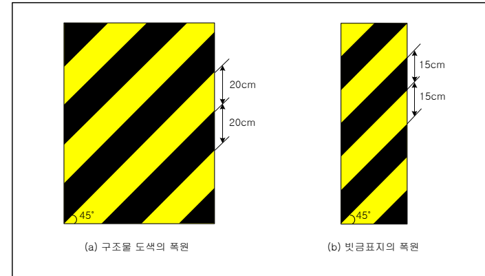
<그림 5.3> 구조물 도색 및 빗금표지의 폭원
