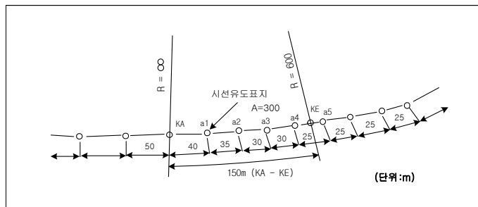
<그림 2.7> 시선유도표지의 설치 (클로소이드구간 사례 1)
