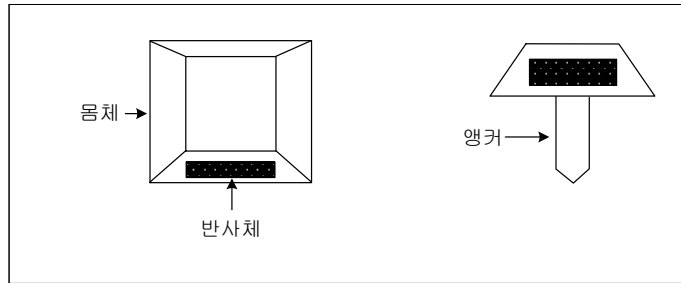
<그림 4.1> 표지병의 구성 요소
