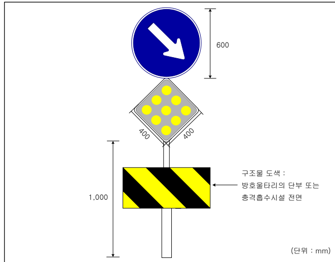
<그림 5.11> 시인성 증진을 위한 관련 시설의 설치
