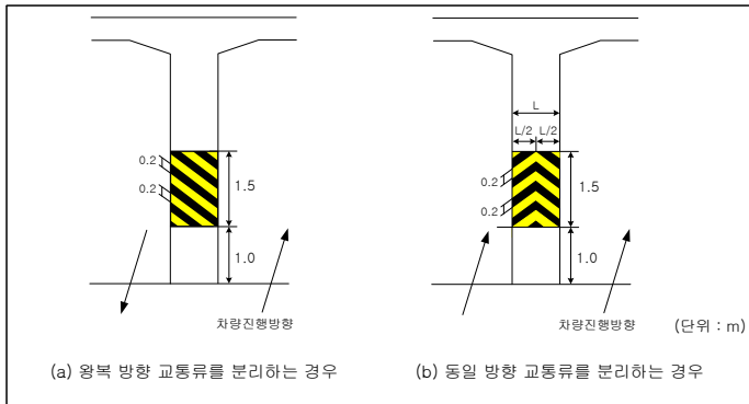
<그림 5.21> 기초가 없는 지하차도의 기둥
