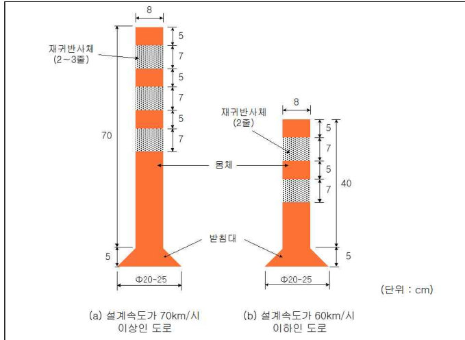
<그림 5.6> 시선유도봉의 형상
