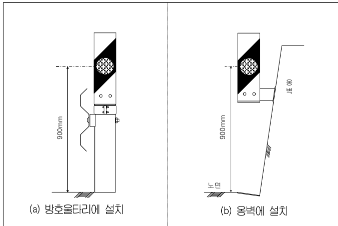
<그림 2.3> 방호울타리, 옹벽에서의 설치 예(각형)
