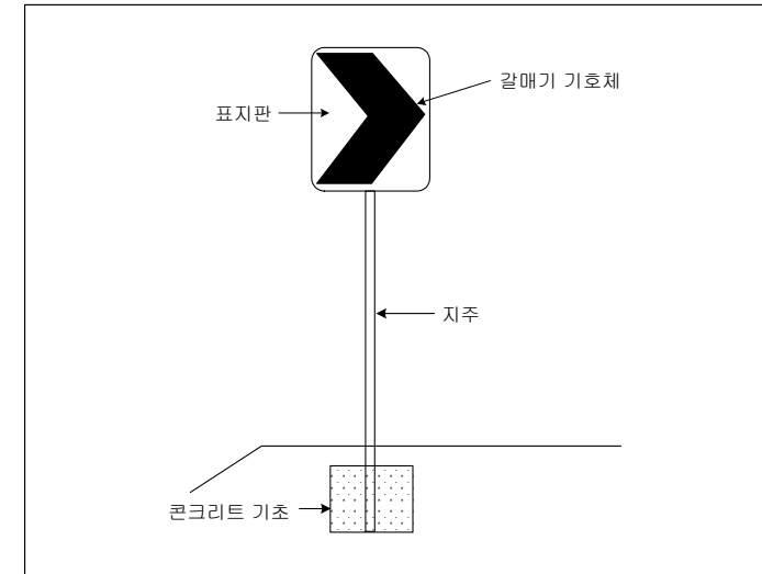
<그림 3.1> 갈매기표지의 구성 요소
