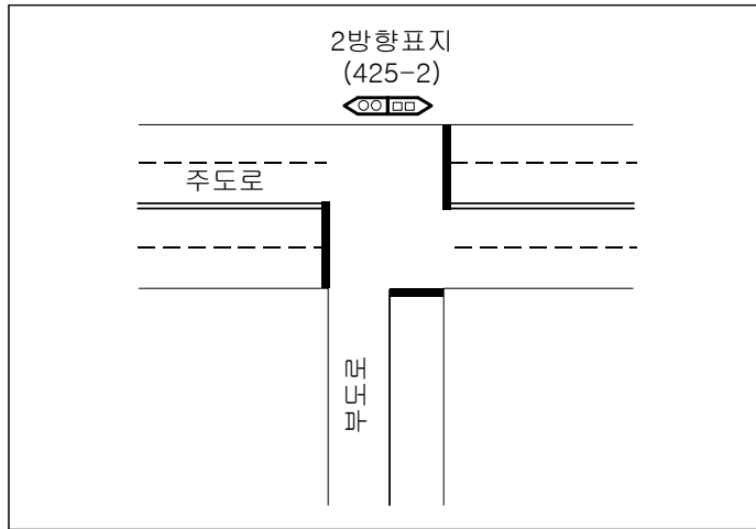
〈그림 5.31〉 3지 교차로의 시선유도 시설 설치
