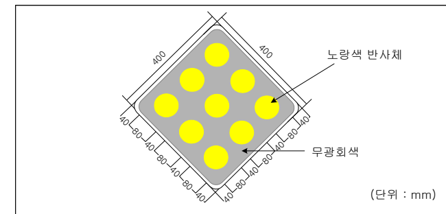
<그림 5.1> 장애물 표적표지의 제원
