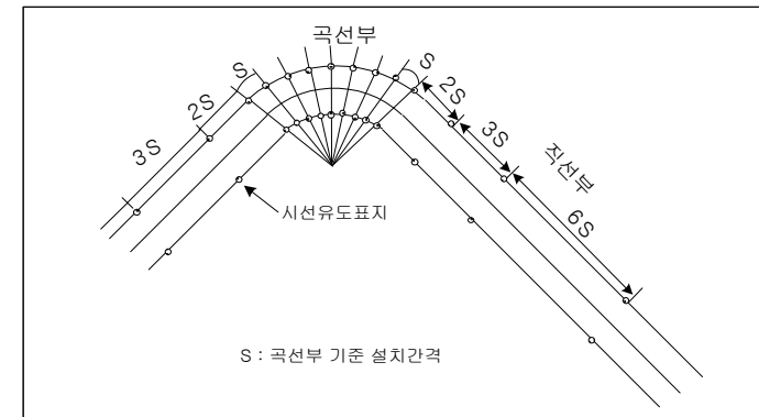
<그림 2.6> 시선유도표지 설치 간격(직선-원곡선 연결구간)
