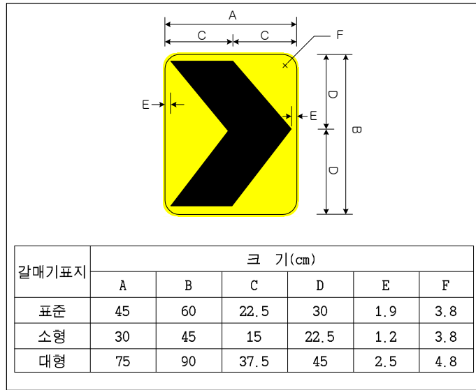
<그림 3.2> 갈매기표지의 크기
