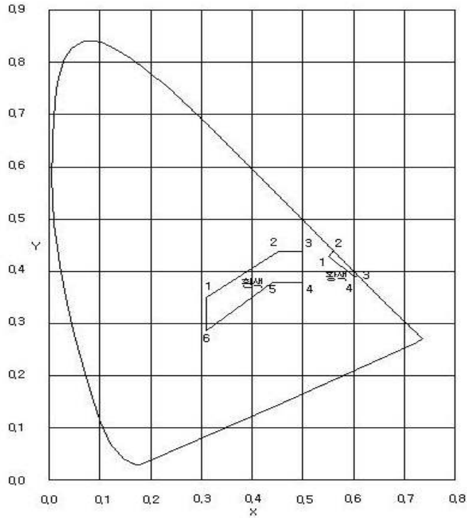
<그림 4.2> 표준색도 좌표
